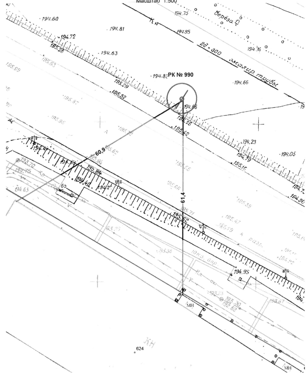
ПОДРОБНАЯ КАРТА № 990 размещения рекламной конструкции по адресу: г. Пенза, ФАД М-5, направлении из Челябинска на Москву, между километровыми указателями 1254-1255, размером 3,0х6,0 Щитовая конструкция Масштаб 1:500
